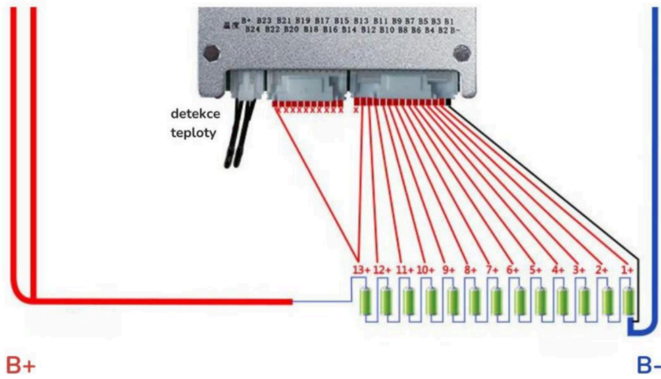
Obr. 15 schéma zapojení 13 stringových bateríí
