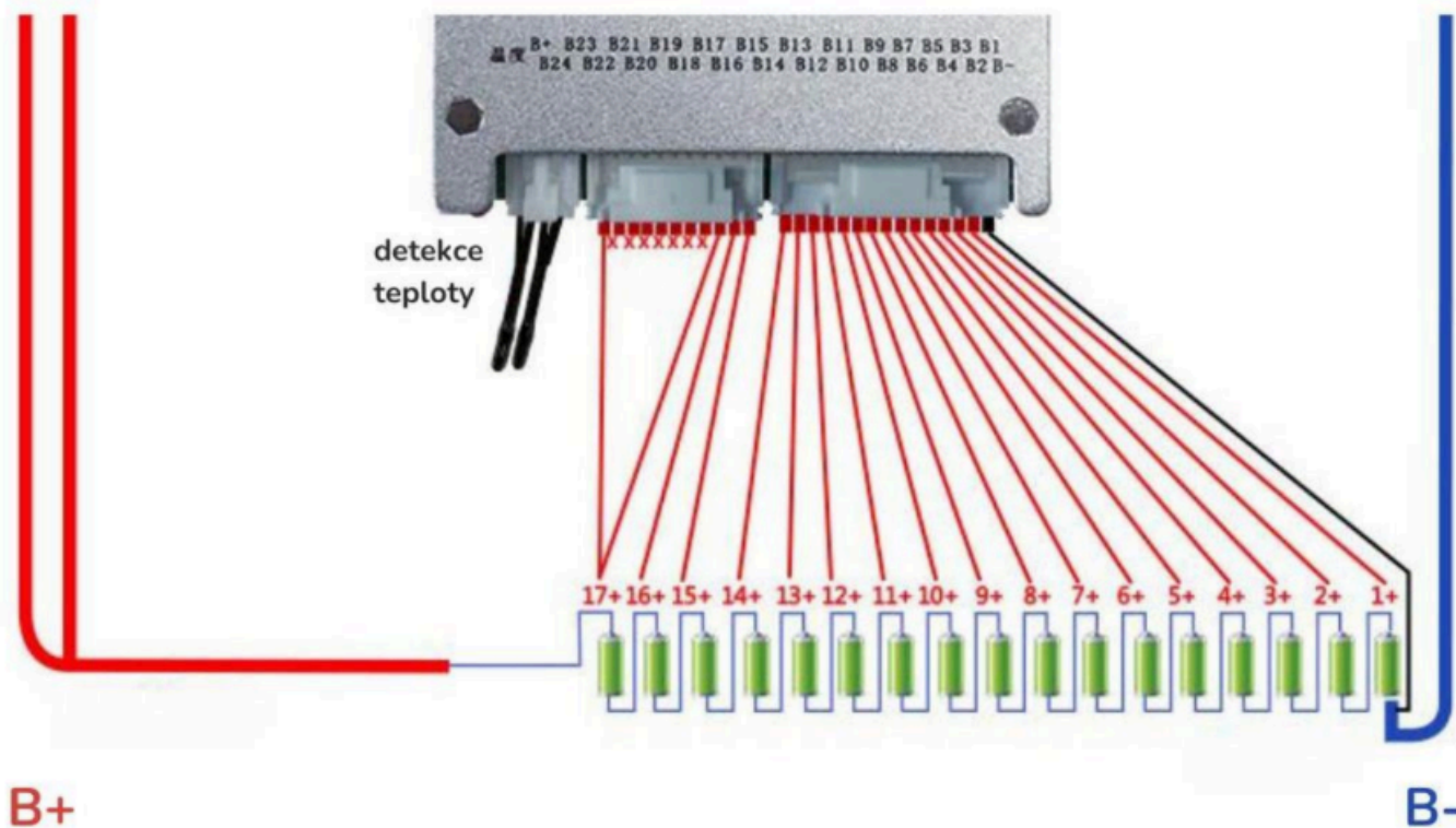
Obr. 14 schéma zapojení 17 stringových bateríí
