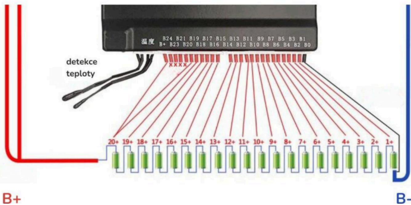
Obr. 9 schéma zapojení 20 stringových baterií
