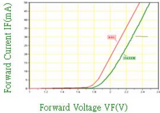
IF-VF (Ta=25°C)
