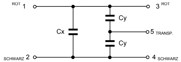
Schéma zapojení
