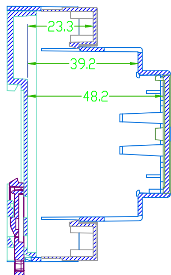
SEC A-A
