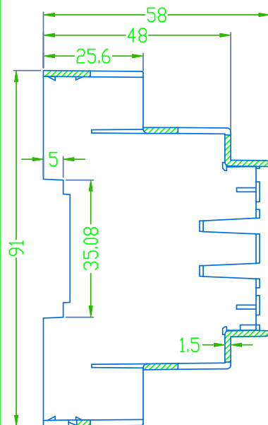
SEC A-A
