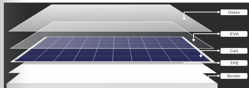
剖面图
