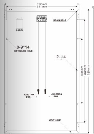
背面图
